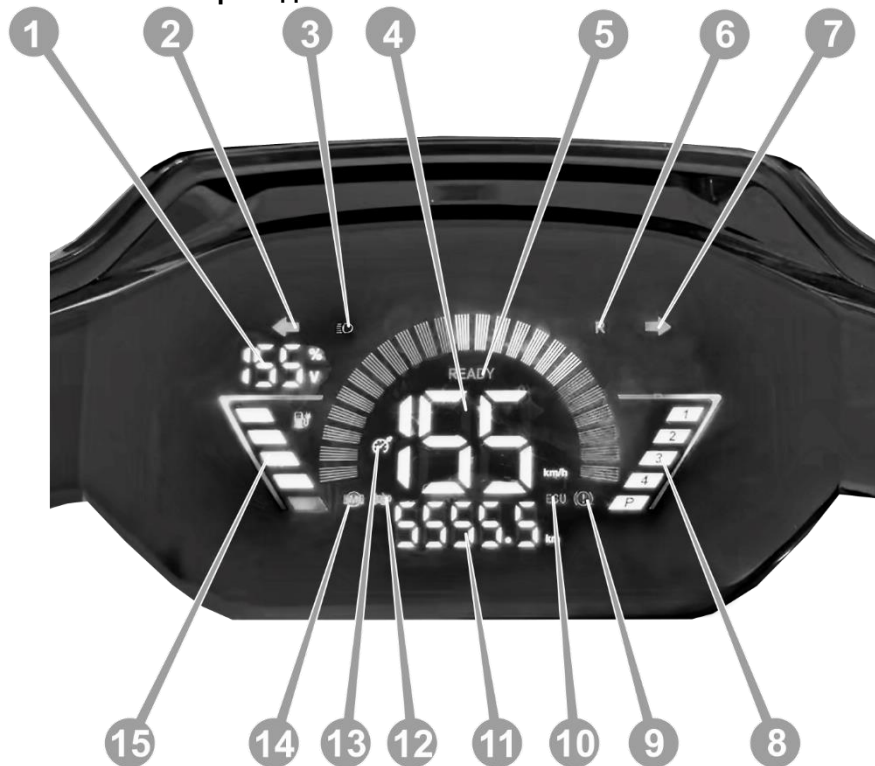
Рисунок 2.1. Панель приладів моделей електроскутера SP1500E-4
