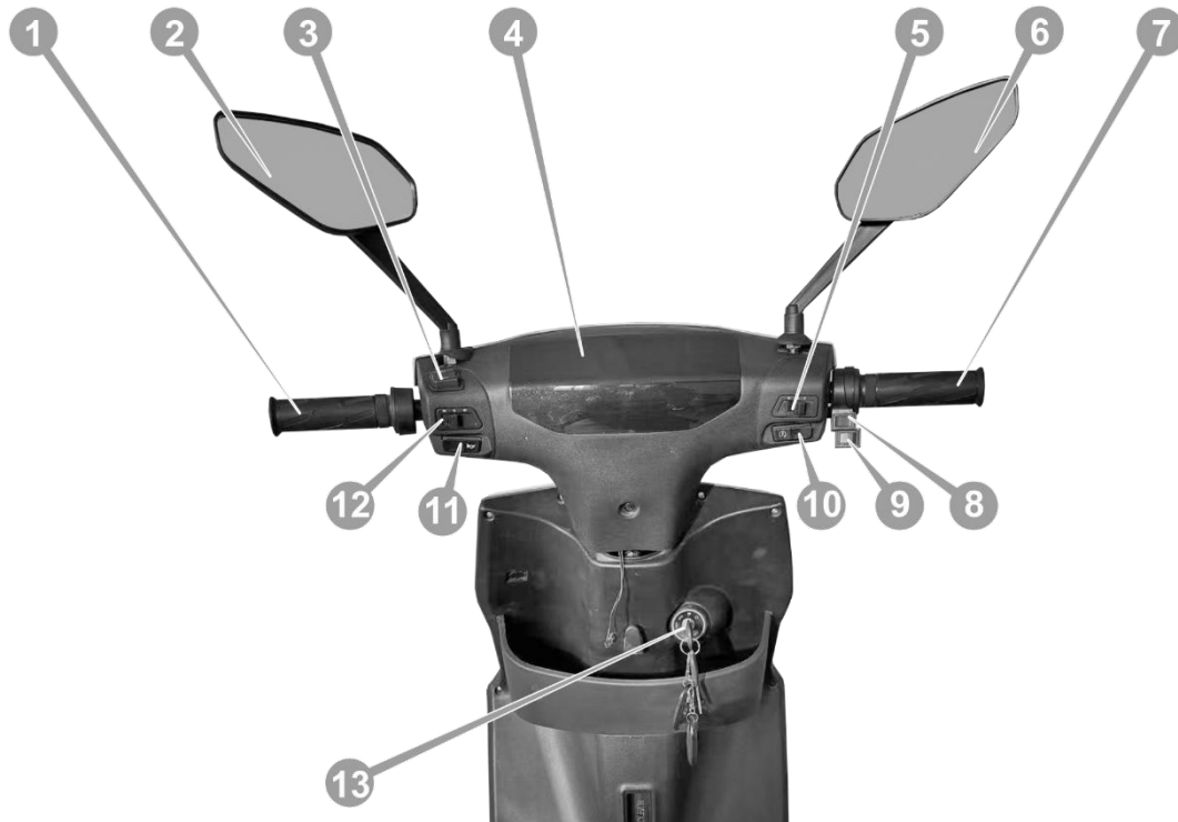
Рисунок 2.3. Кермо електроскутера, блоки керування на кермі
