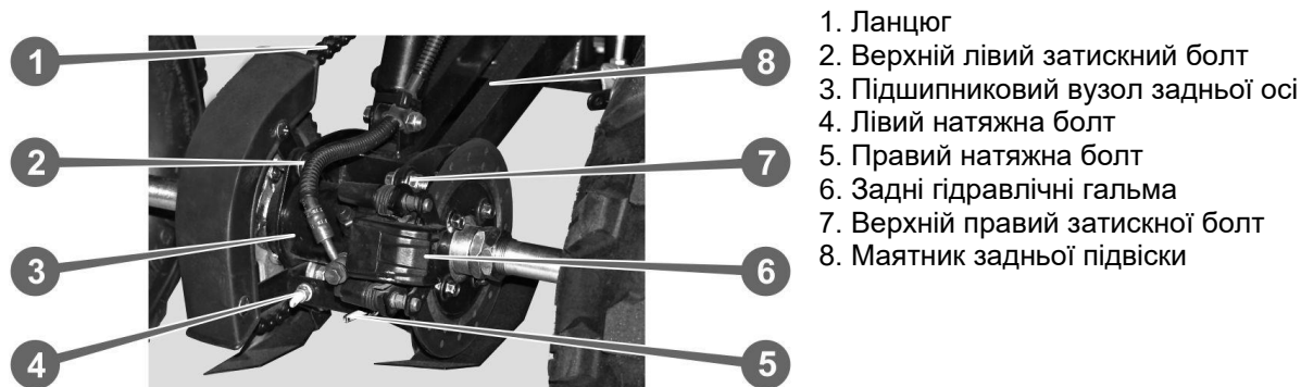
Рисунок 7.8. Механізм натягу ланцюга.
