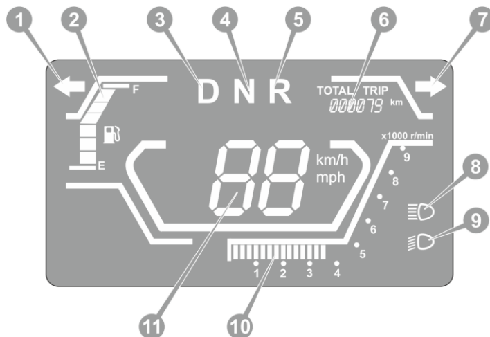
Рисунок 3.3 Панель приладів моделі SP200-10 (2026)
