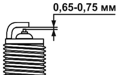
Рисунок 7.5. Свічка запалювання, регулювання зазору
