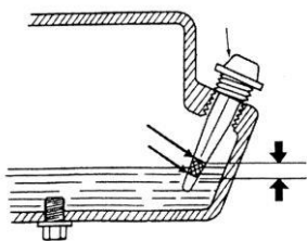
Рисунок 7.4. Перевірка рівня мастила в двигуні
