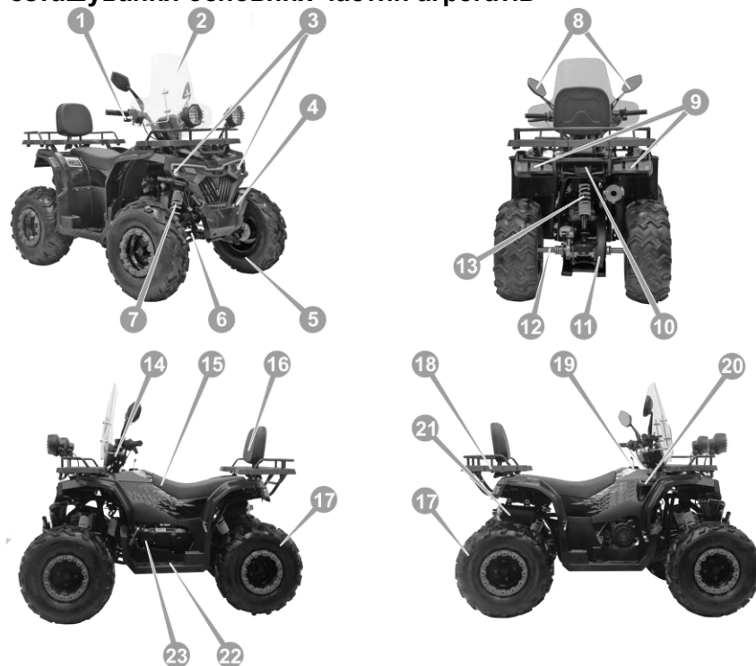
Рисунок 3.1.1 Розташування вузлів та агрегатів моделей SP200-10 (2026)
