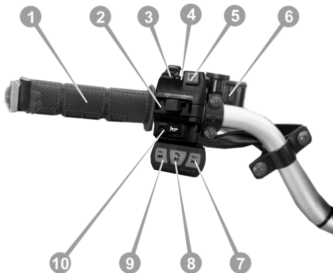
Рисунок 3.4. Блок перемикачів лівий
