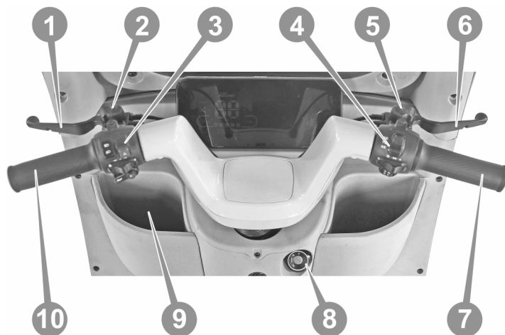
Рисунок 3.2. Кермо електротрицикла
