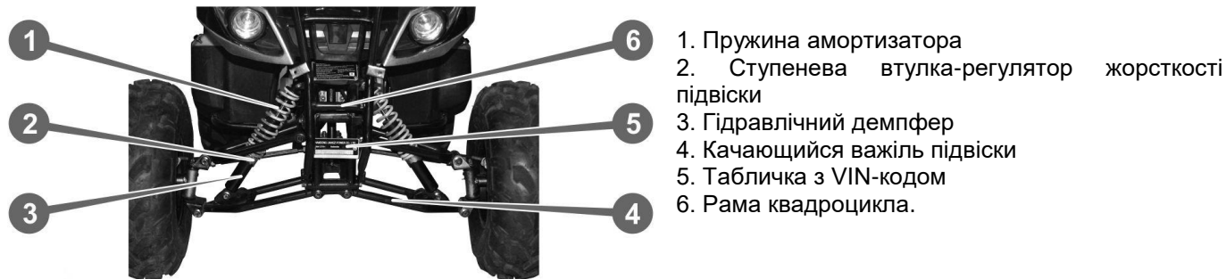
Рисунок 7.7. Передній міст
