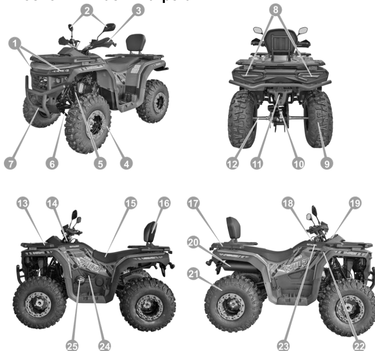
Рисунок 3.1. Розташування вузлів та агрегатів моделей SPARK WILD 200, SPARK WILD 200SE
