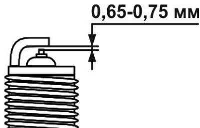
Рисунок 7.4. Свічка запалювання, регулювання зазору
