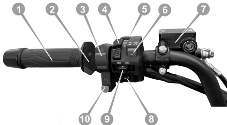
Рисунок 3.4. Блок перемикачів лівий
