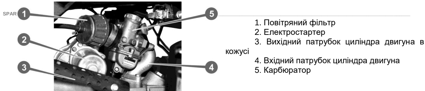
Рисунок 7.5. Повітряний фільтр, карбюратор
