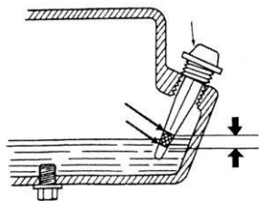
Рисунок 7.3. Перевірка рівня мастила в двигуні
