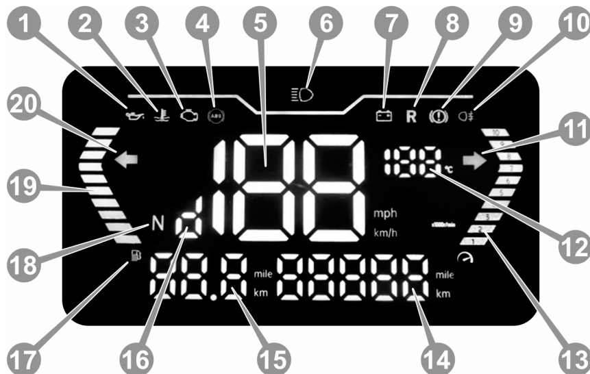
Рисунок 3.3. Панель приладів
