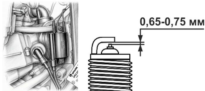
Рисунок 6.4. Свічка запалювання, регулювання зазору
