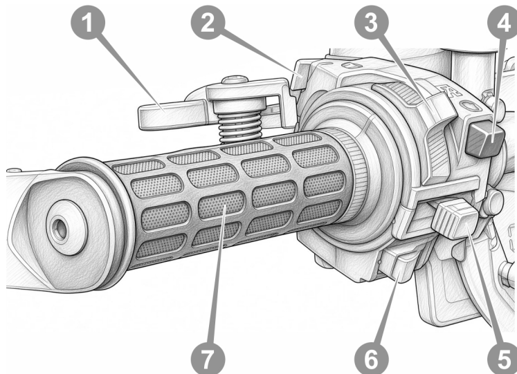
Рисунок 3.4. Блок перемикачів на кермі зліва.
