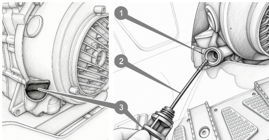
Рисунок 6.2. Перевірка рівня мастила в двигуні
