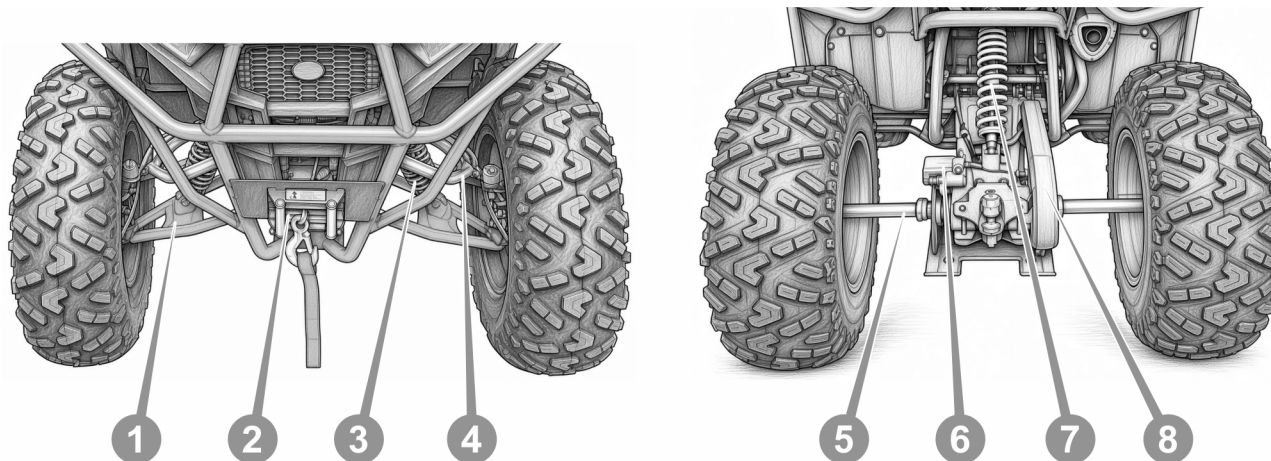
Рисунок 6.7. Ходова частина
