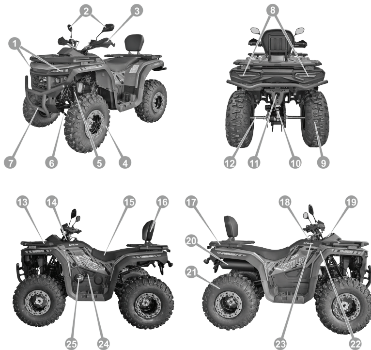
Рисунок 3.1. Розташування основних вузлів та агрегатів
