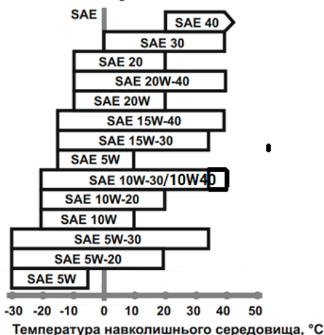
Рисунок 4. Залежність густини мастила від температури сезону.
