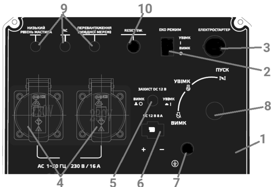
Рисунок 2. Панель керування.
