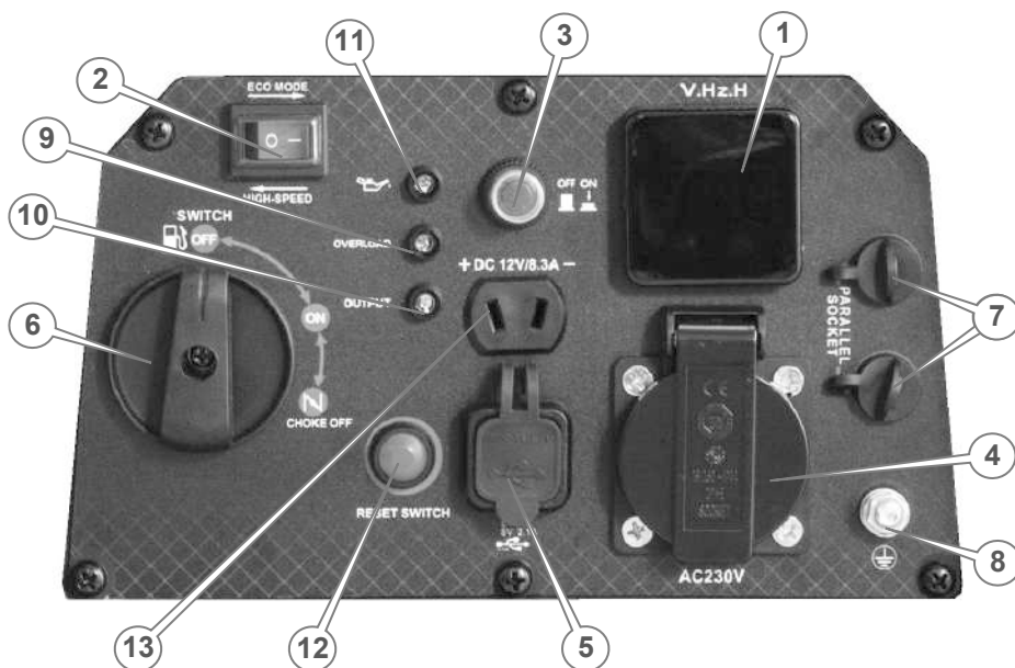
Рисунок 2. Панель керування моделі «IG 3.5bse».
