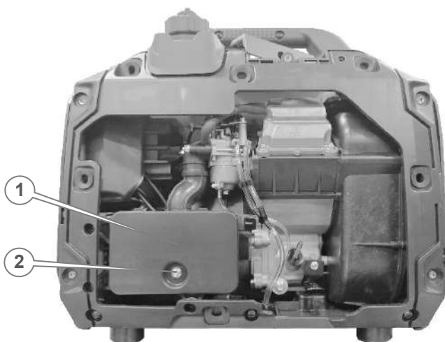
Рисунок 6. Схема розташування повітряного фільтра
