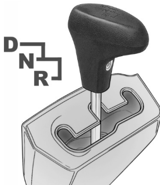
Рисунок 3.6. Важіль вибору напрямку руху
