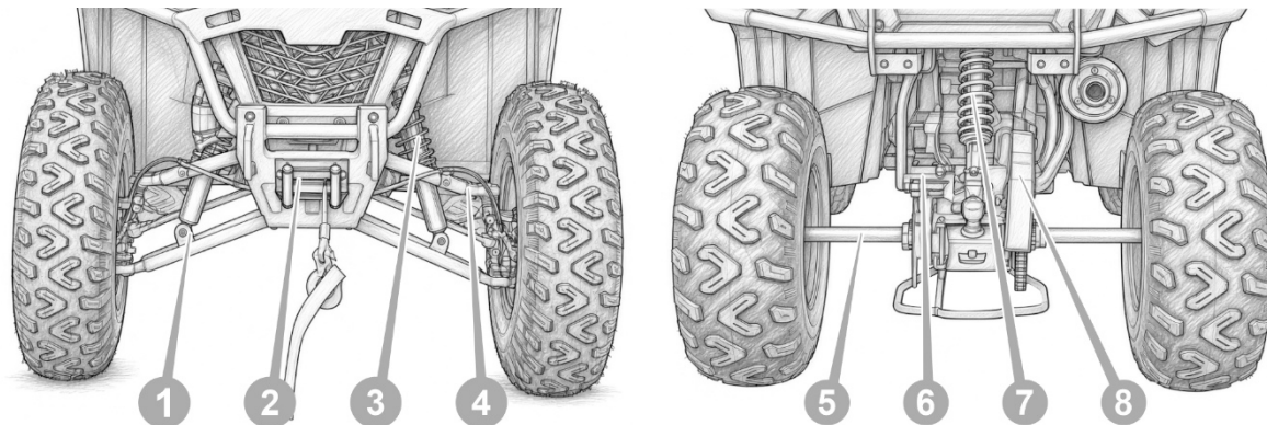
Рисунок 6.8. Ходова частина
