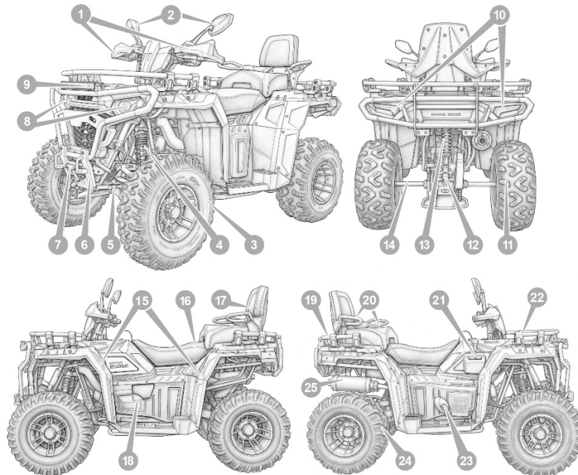
Рисунок 3.1. Розташування основних вузлів та агрегатів
