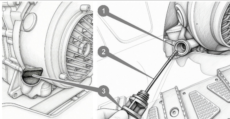
Рисунок 6.3. Перевірка рівня мастила в двигуні
