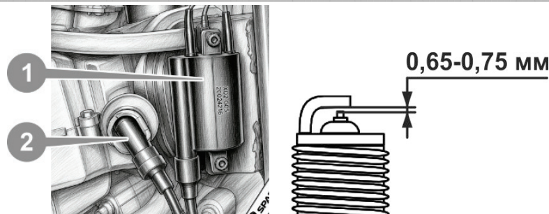
Рисунок 6.5. Свічка запалювання, регулювання зазору
