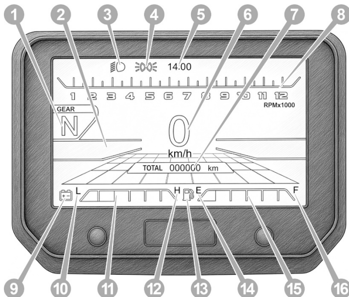
Рисунок 3.3. Панель приладів
