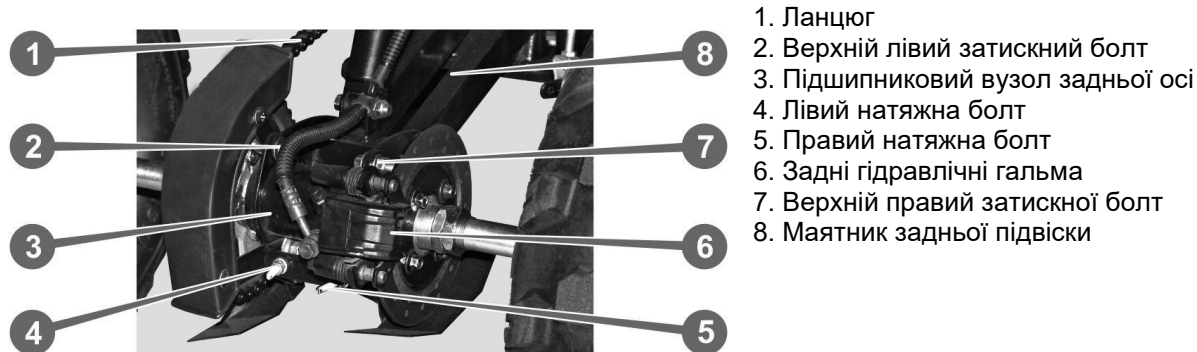
Рисунок 7.8. Механізм натягу ланцюга.
