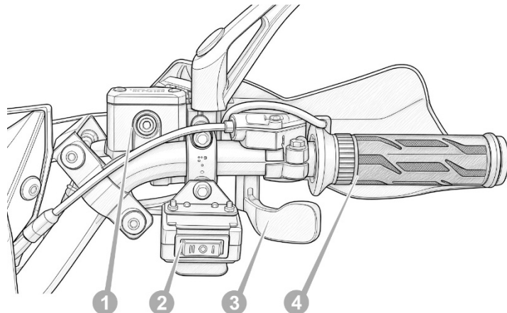
Рисунок 3.5. Блок перемикачів на кермі справа
