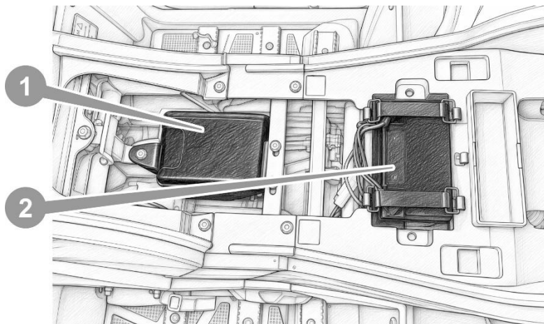
Рисунок 6.6. Повітряний фільтр, акумулятор. Вид зверху зі знятим сидінням квадроцикла
