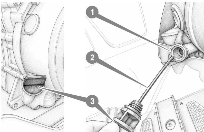
Рисунок 6.3. Перевірка рівня мастила в двигуні
