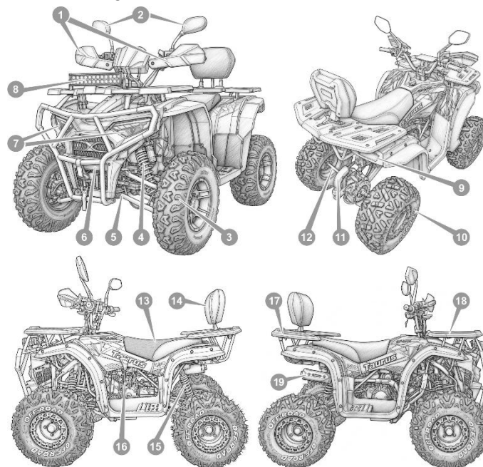
Рисунок 3.1. Розташування основних вузлів та агрегатів
