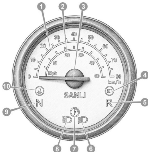
Рисунок 3.3. Панель приладів
