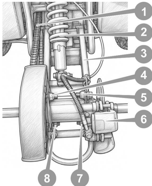
Рисунок 6.7. Механізм натягу ланцюга.
