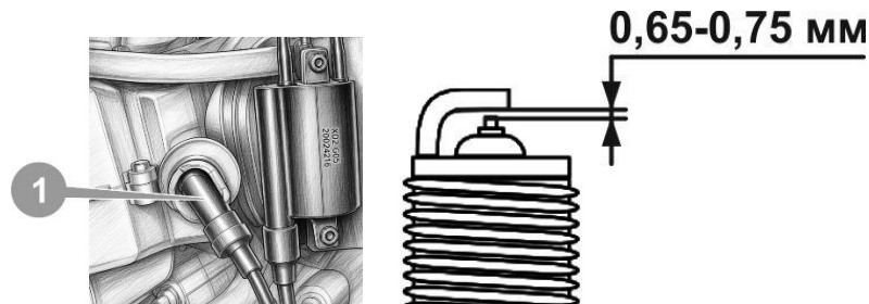
Рисунок 6.5. Свічка запалювання, регулювання зазору
