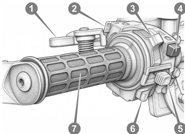
Рисунок 3.4. Блок перемикачів на кермі зліва
