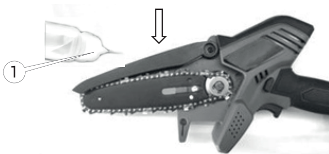
Рисунок 5. Схема змащення напрямної.
