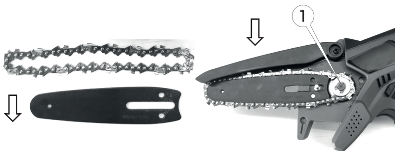
Рисунок 3. Встановлення ланцюга на напрямній.
