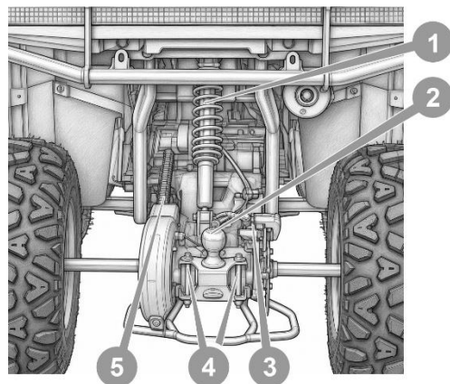
Рисунок 6.7. Механізм натягу ланцюга.
