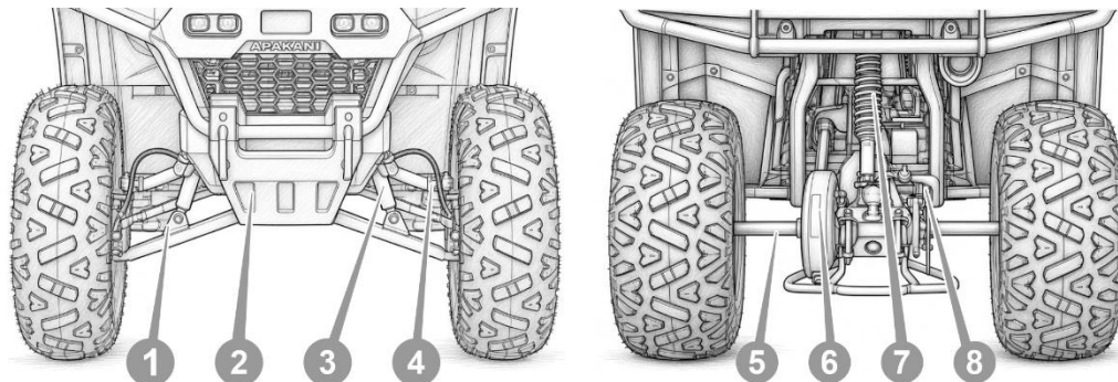
Рисунок 6.8. Ходова частина
