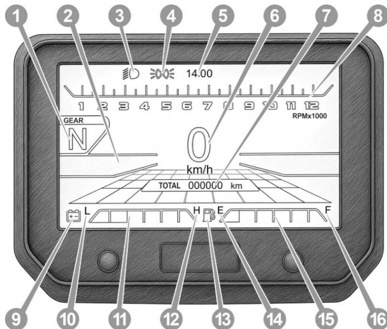
Рисунок 3.3. Панель приладів
