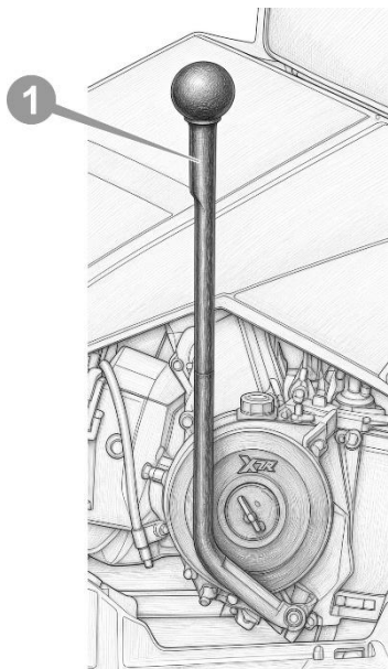
Рисунок 3.6. Важіль вибору напрямку руху
