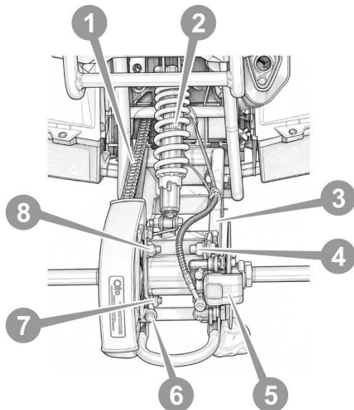
Рисунок 6.7. Механізм натягу ланцюга.
