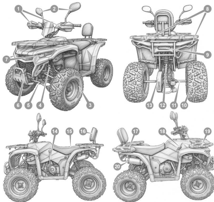
Рисунок 3.1. Розташування основних вузлів та агрегатів
