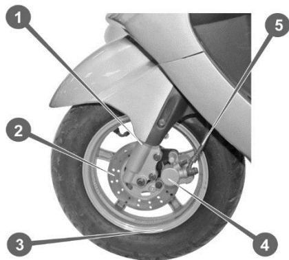
Рис. 5.5. Переднє гальмо
