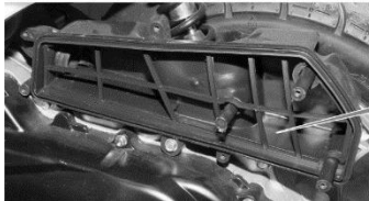
Рисунок 5.3. Повітряний фільтр.
