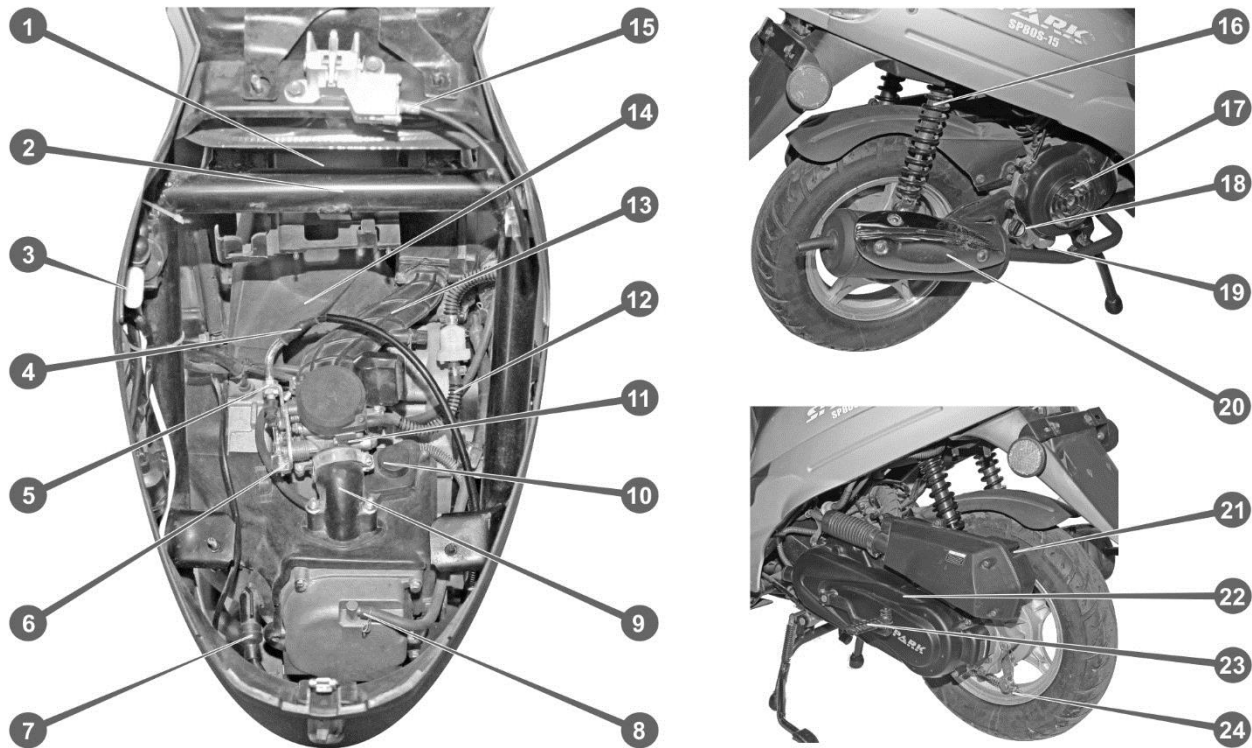
Рис. 3.3. Силовий агрегат 17
