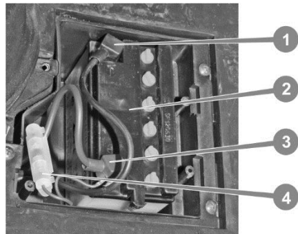
Рис. 5.5 Акумуляторна батарея
