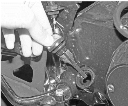
Рис. 5.1. Перевірка рівня мастила в двигуні
