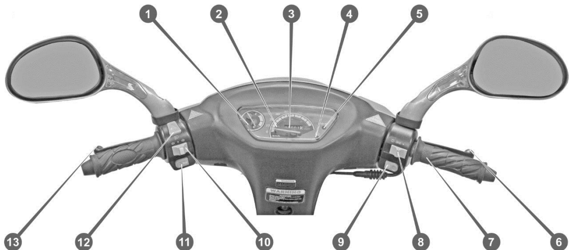
Рис. 3.2. Панель приладів
