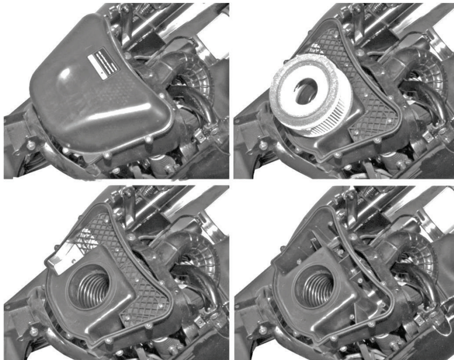
Рис. 6.6. Повітряний фільтр
