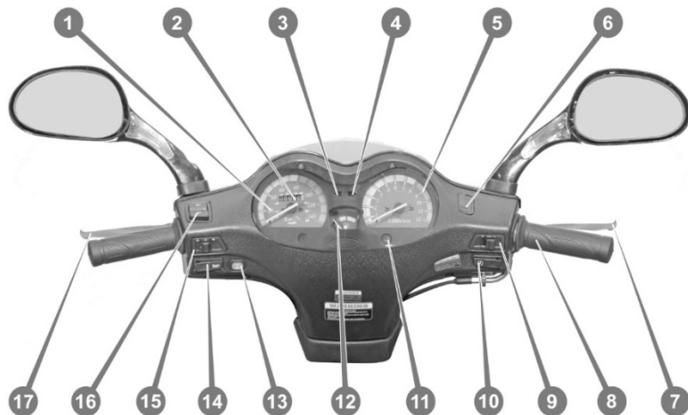
Рис. 3.2. Панель приладів
