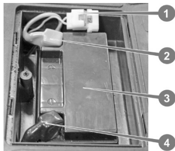
Рис. 5.5. Аккумуляторна батарея
