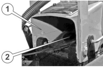
Рисунок 31. – Кріплення керма
