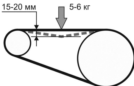
Рисунок 44. – Схема натягу ремня
