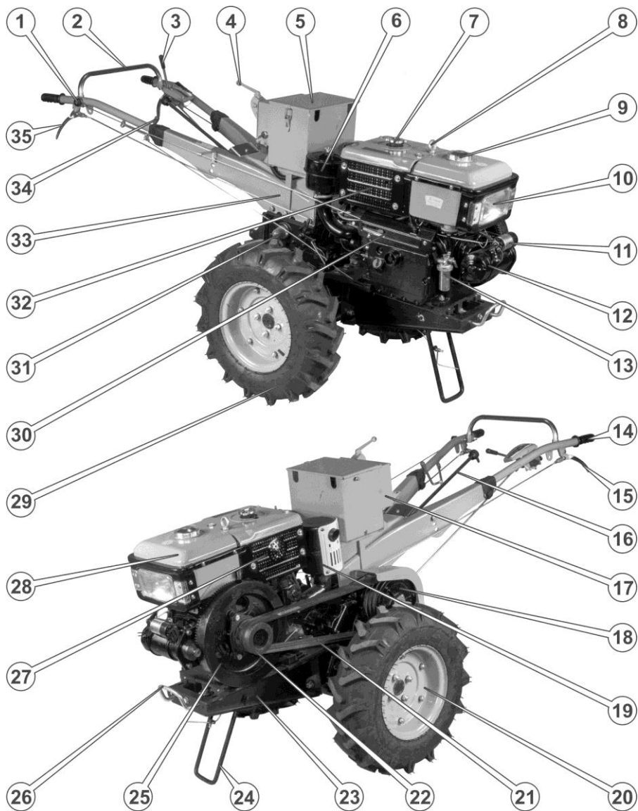
Рисунок 7. – Органи мотоблока МБ 1012Е
