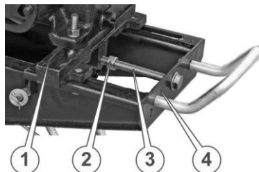
Рисунок 21. – Елементи бампера
