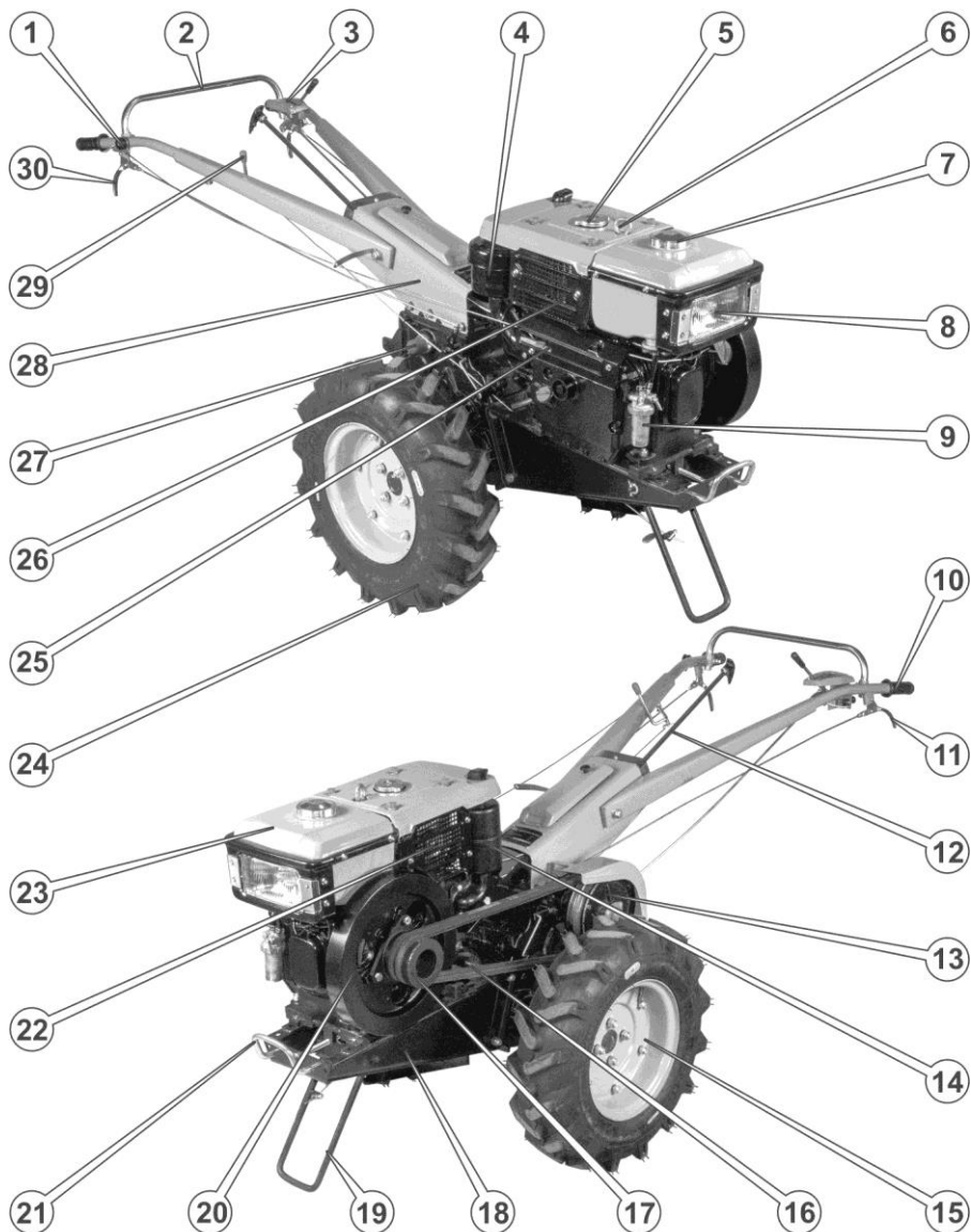
Рисунок 6. – Органи мотоблока МБ 1010
