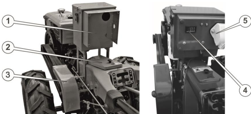
Рисунок 22. – Вид з місця АКБ
