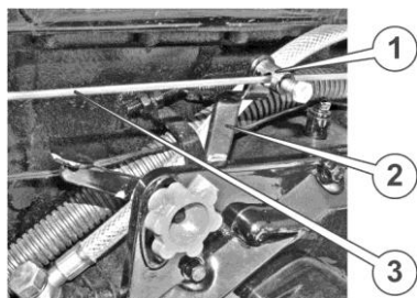
Рисуюнок 29. – Тяга подачі палива
