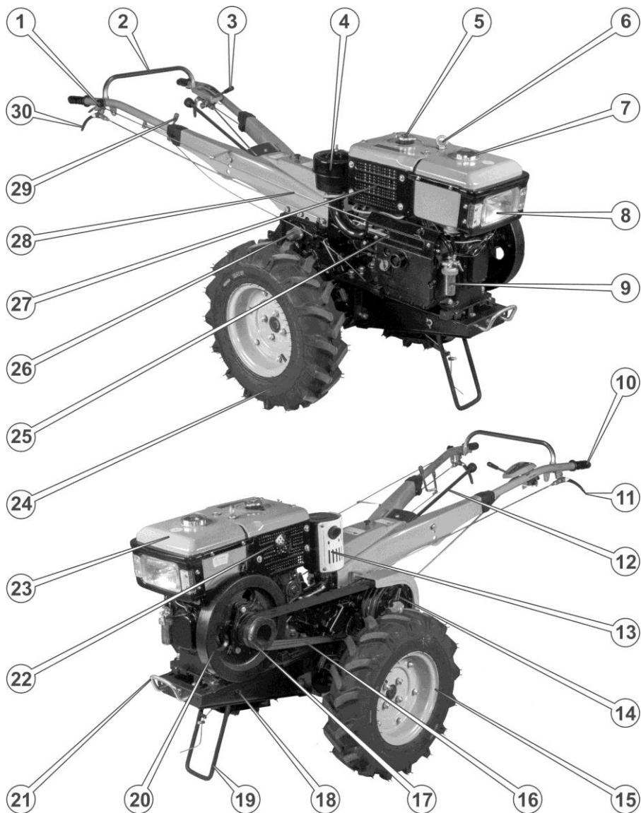
Рисунок 9. – Органи мотоблока МБ 1012
