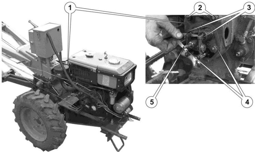
Рисунок 38. – Відкрита головка циліндра
