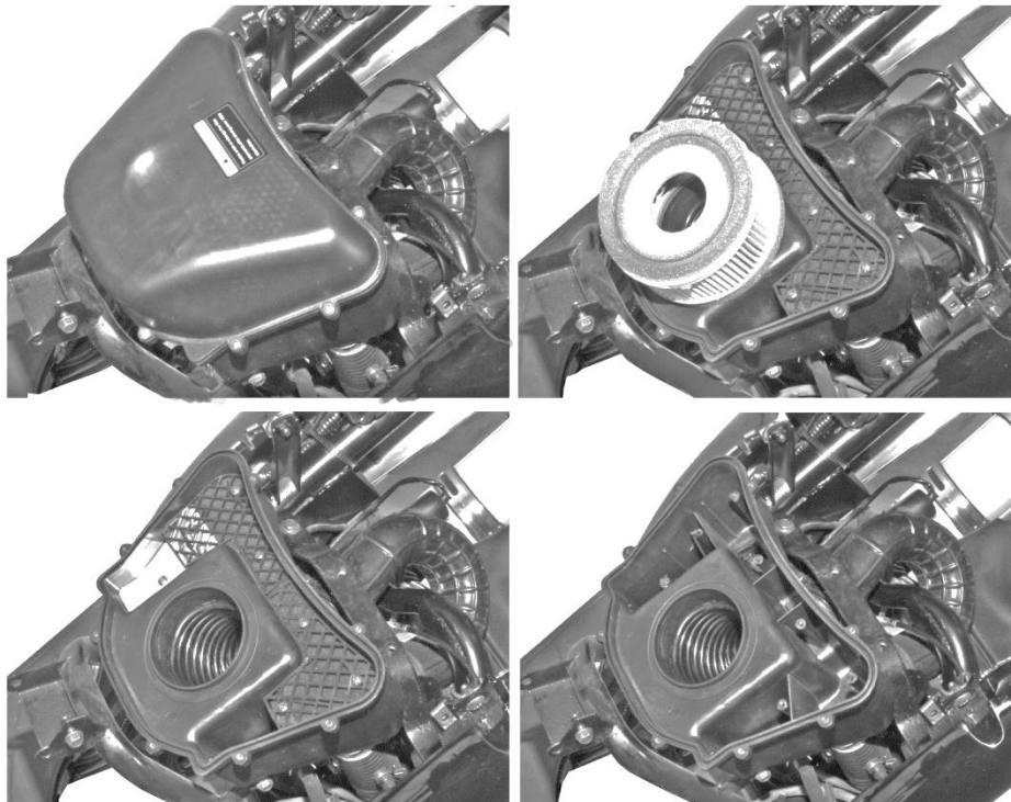
Рис. 5.6. Повітряний фільтр
