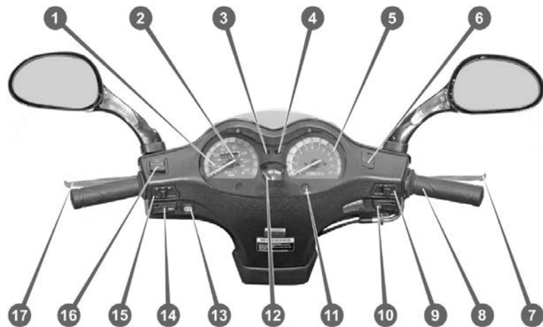
Рис. 3.2. Панель приладів
