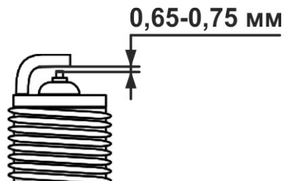
Рис. 5.5. Свіча запалювання, регулювання зазору
