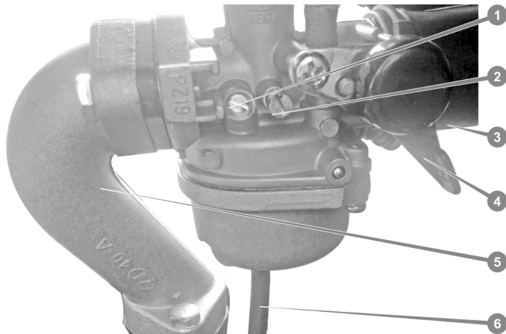
Рисунок 7. Карбюратор
