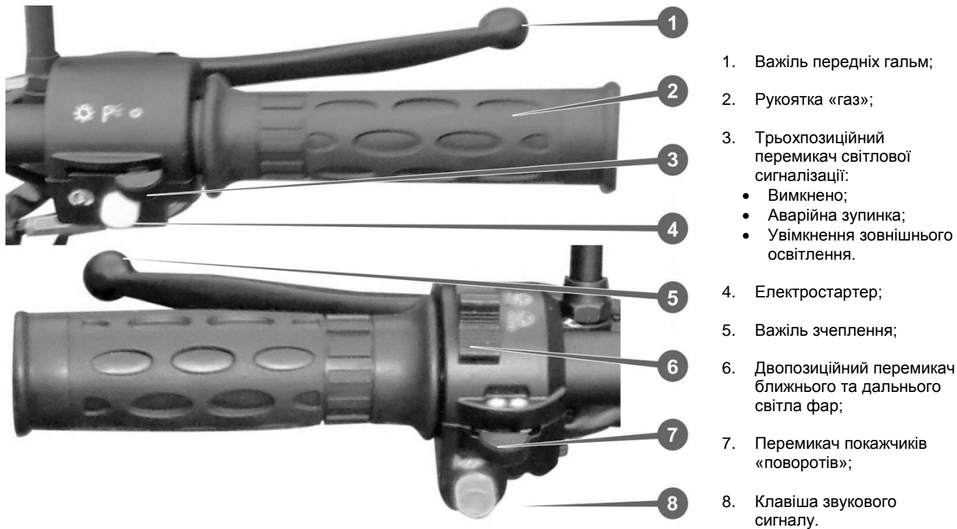
Рисунок 4. Права та ліва рукоятки керма
