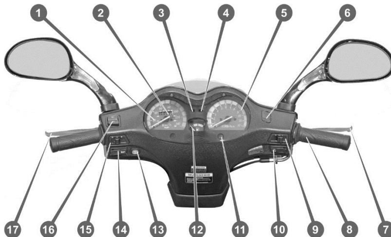
Рис. 3.2. Панель приладів
