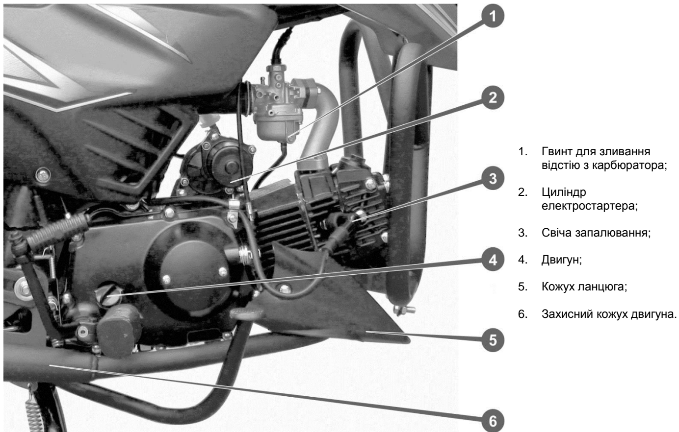
Рисунок 4. Вид двигуна праворуч
