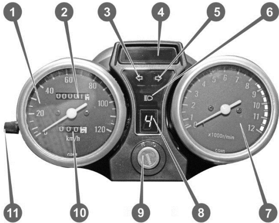
Рисунок. 2. Панель приладів
