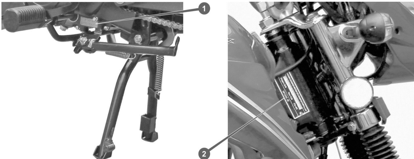
Рисунок 6. Серійні номери
