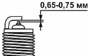
Рис. 14. Свічка запалювання, регулювання зазору.
