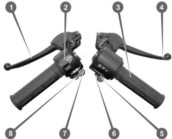
Рисунок. 3. Блоки перемикачів
