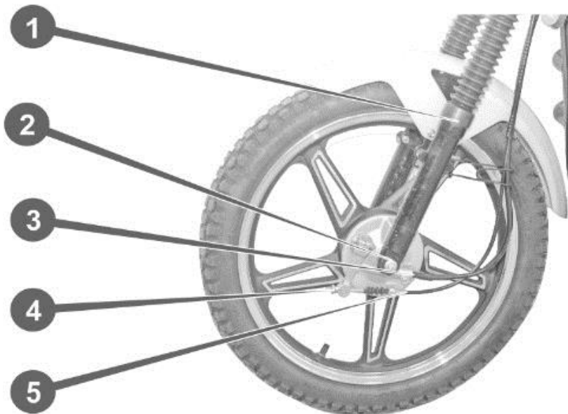
Рисунок 17. Переднє гальмо
