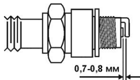
Рис. 16. – Необхідний зазор свічки запалювання
