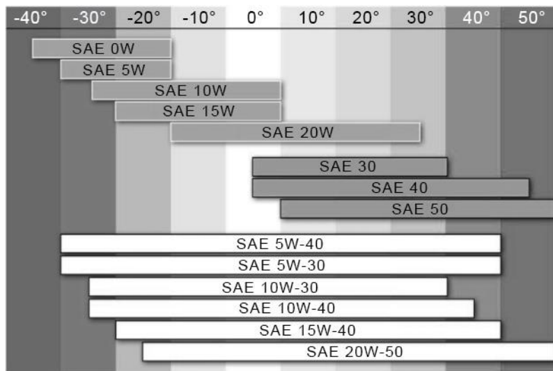
Рис. 12. – Температурно-діапазонний графік в'язкості моторного мастила
