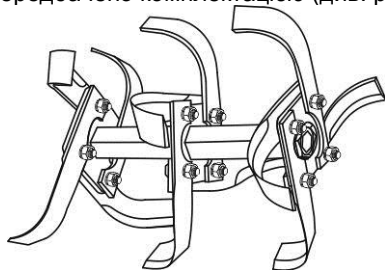
Рис. 10. – Ґрунтофреза у зборі
