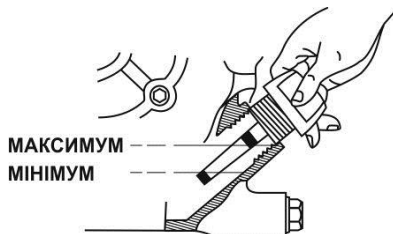
Рис. 11. – Пробка-щуп картера двигуна
