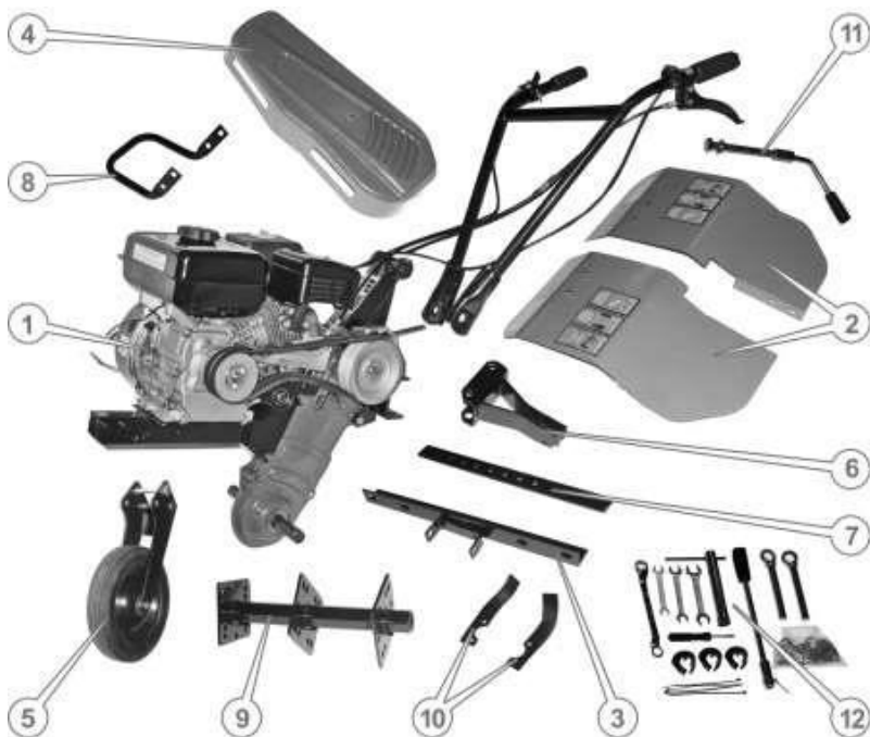
Рис. 2. – Розгорнута комплектація мотоблоку
