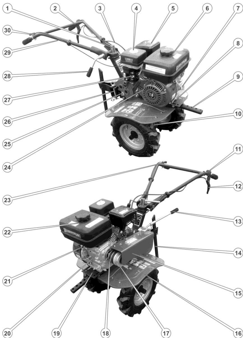
Рис. 3. – Елементи мотоблока
