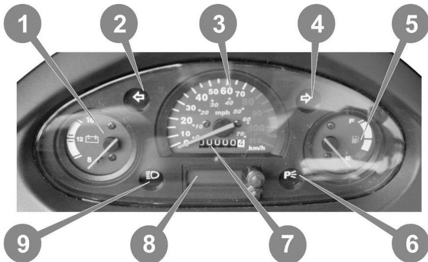
Рис. 3.3. Приладова панель
