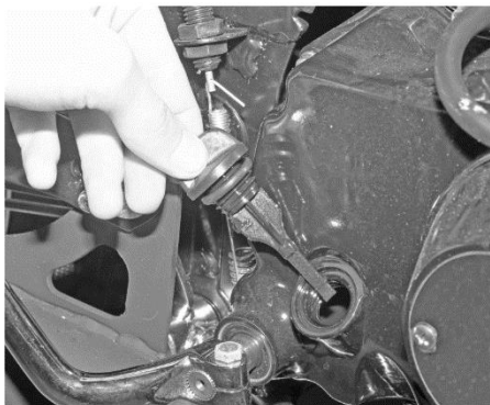
Рис. 5.1. Перевірка рівня мастила у двигуні Для перевірки рівня мастила необхідно пробку-щуп (див. рис. 5.2.). Вставити в заливну горловину, при цьому не закру-
