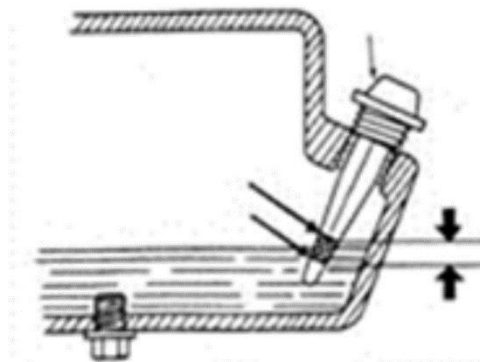
Рис. 5.1. Перевірка рівня мастила у двигуні Для перевірки рівня мастила необхідно пробку-щуп (див. рис. 5.2.). Вставити в заливну горловину, при цьому не закру-
