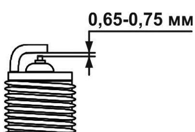
Рисунок 5.5. Свічка запалювання, регулювання зазору
