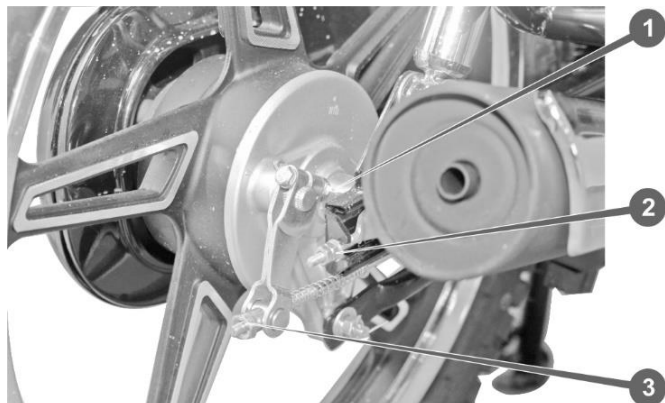
Рисунок 19. Заднє гальмо
