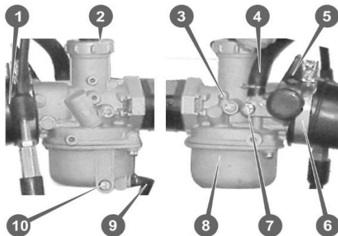
Рис. 16. Карбюратор
