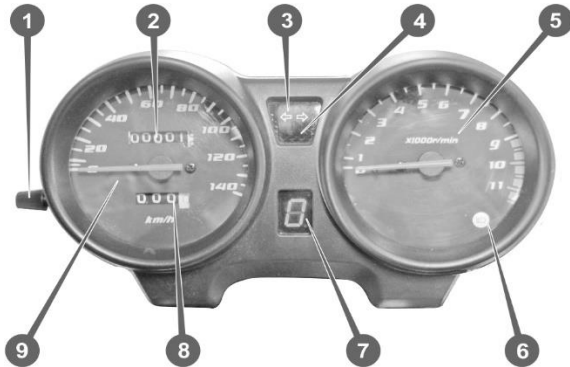
Рис. 3. Панель приладів
