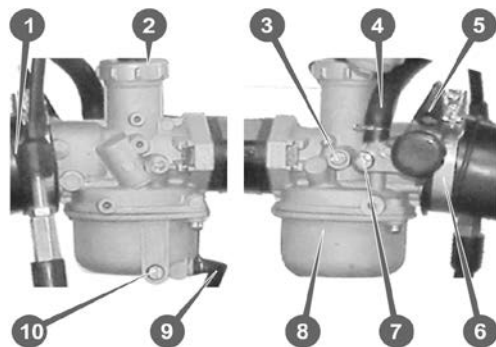
Рис. 15.1. Карбюратор
