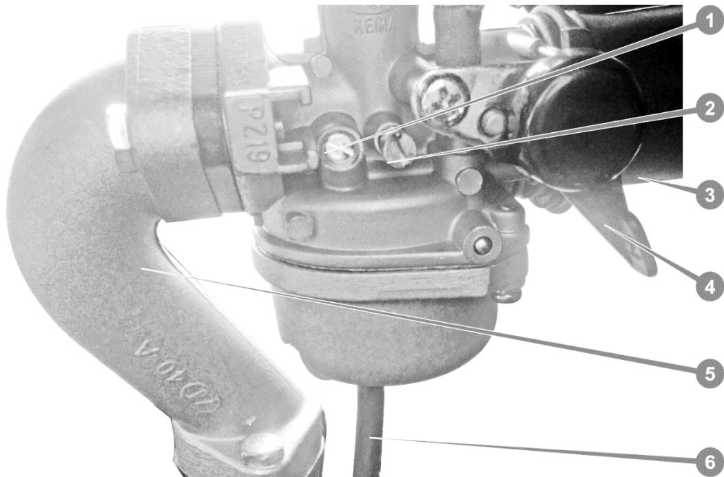
Рисунок 7. Карбюратор
