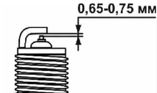
Рис. 14. Свічка запалювання, регулювання зазору.
