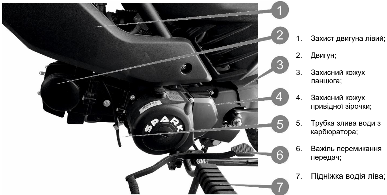
Рис. 5. Вид двигуна ліворуч
