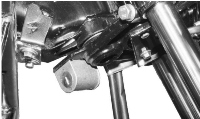
Рис. 10. Замок блокування керма
