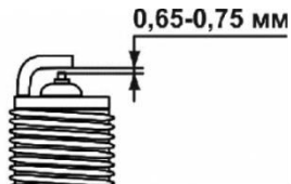
Рис. 15. Свічка запалювання, регулювання зазору.
