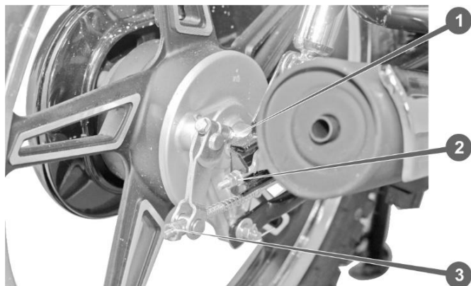
Рис. 19. Задня гальмівна система
