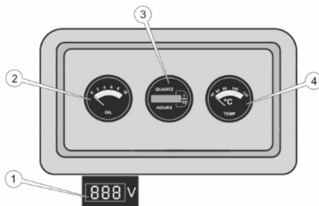
Рисунок 3.7. Панель приладів
