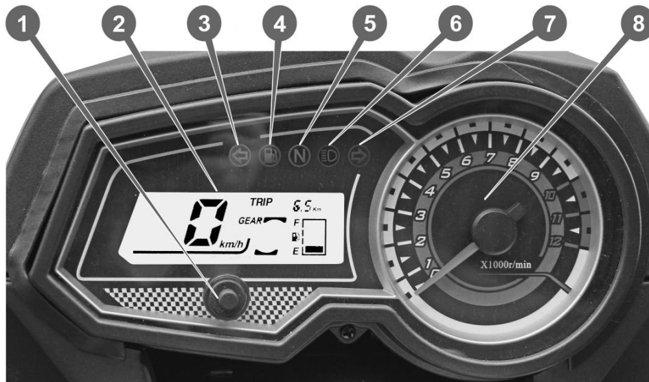
Рис. 3.2. Приладова панель
