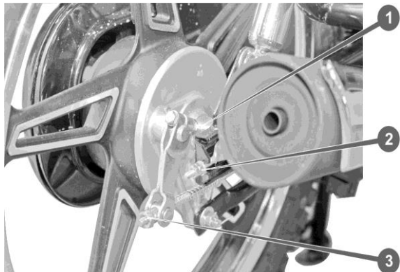
Рис. 6.10 Колесо заднє
