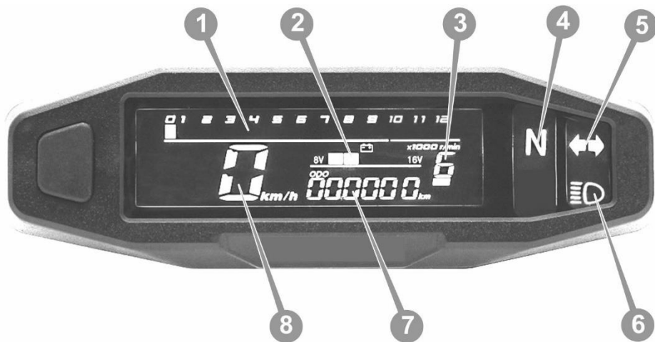
Рисунок 2. Приладова панель
