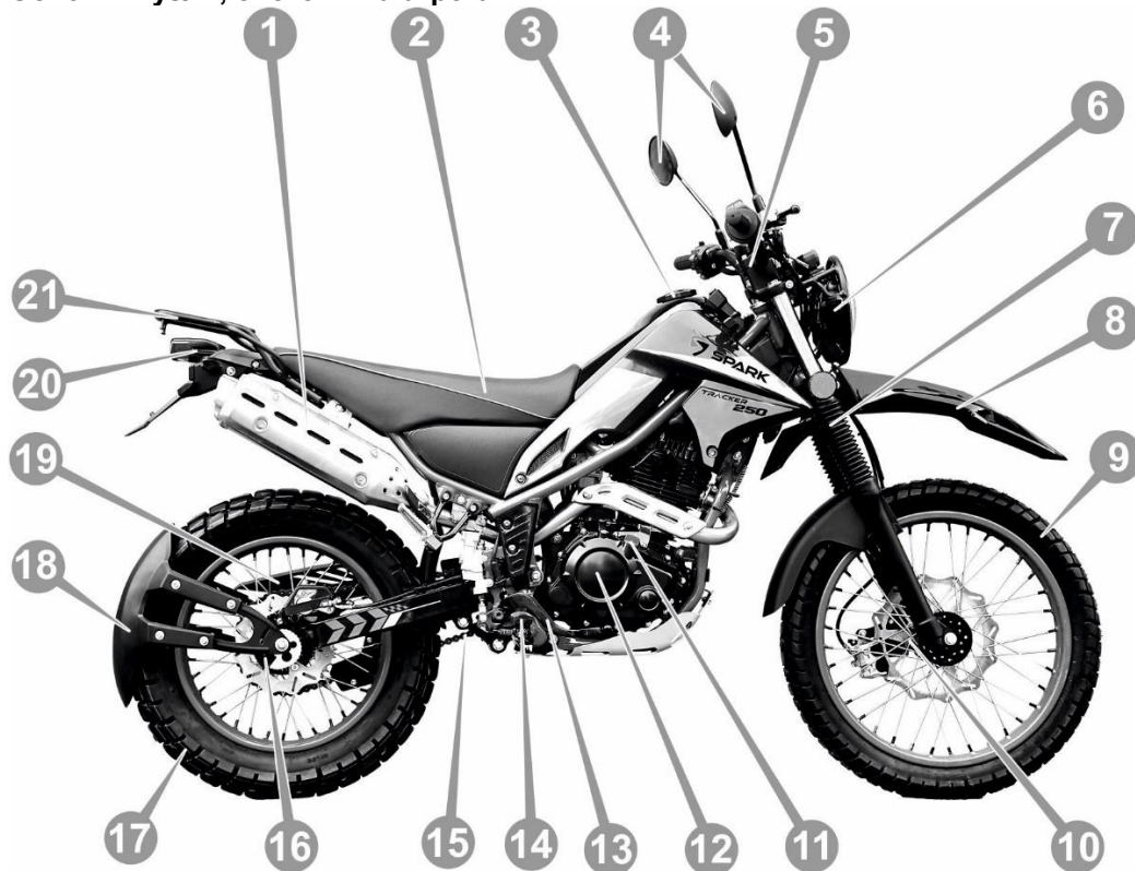
Рисунок 1. Мотоцикл, вид праворуч
