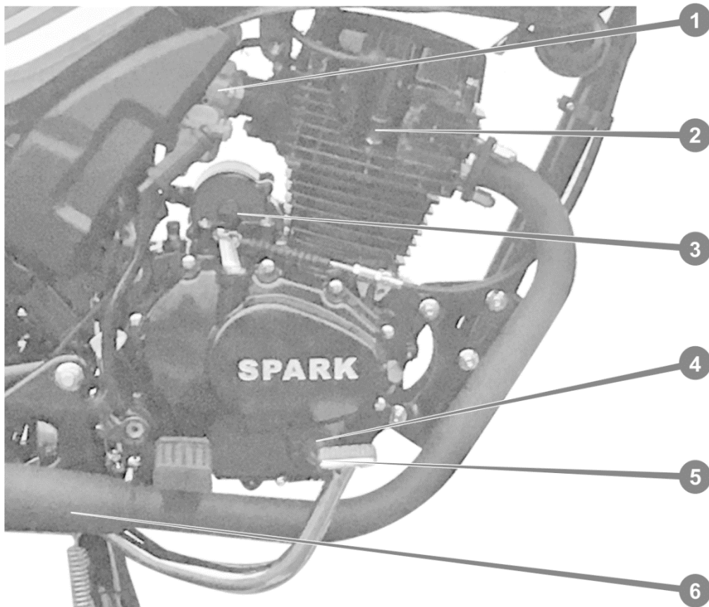
Рисунок 3.5. Вид двигуна праворуч
