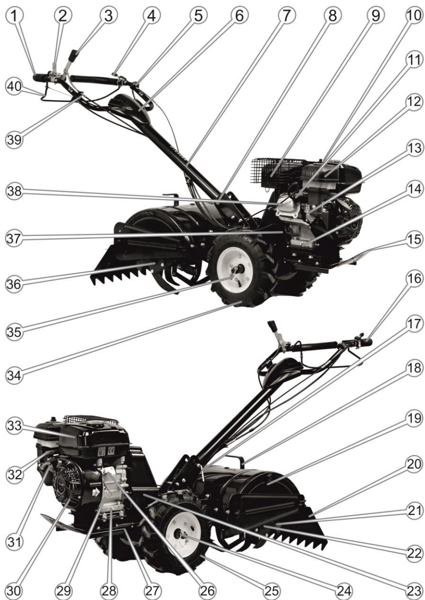
Рисунок 1.1. Елементи мотоблока
