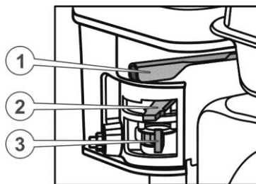
Рисунок 4.13. Регулювальні елементи карбюратора
