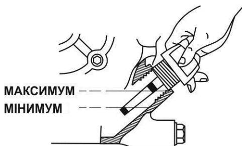
Рисунок 4.10. Пробка-щуп картера двигуна
