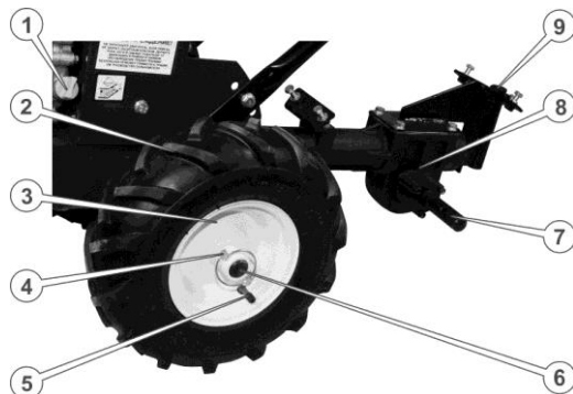
Рисунок 4.4. Ліва частина мотоблока
