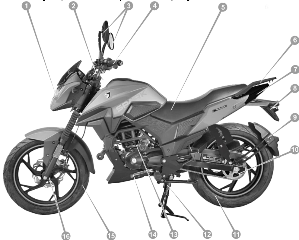
Рисунок 3.1. Мотоцикл SPARK SP20R-32
