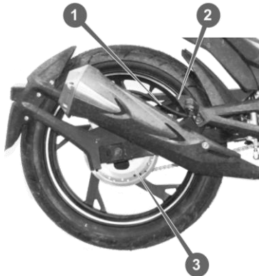
Рис. 6.10. Колесо заднє
