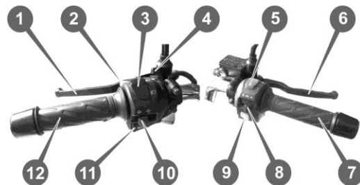
Рисунок 3.4. Блоки перемикачей
