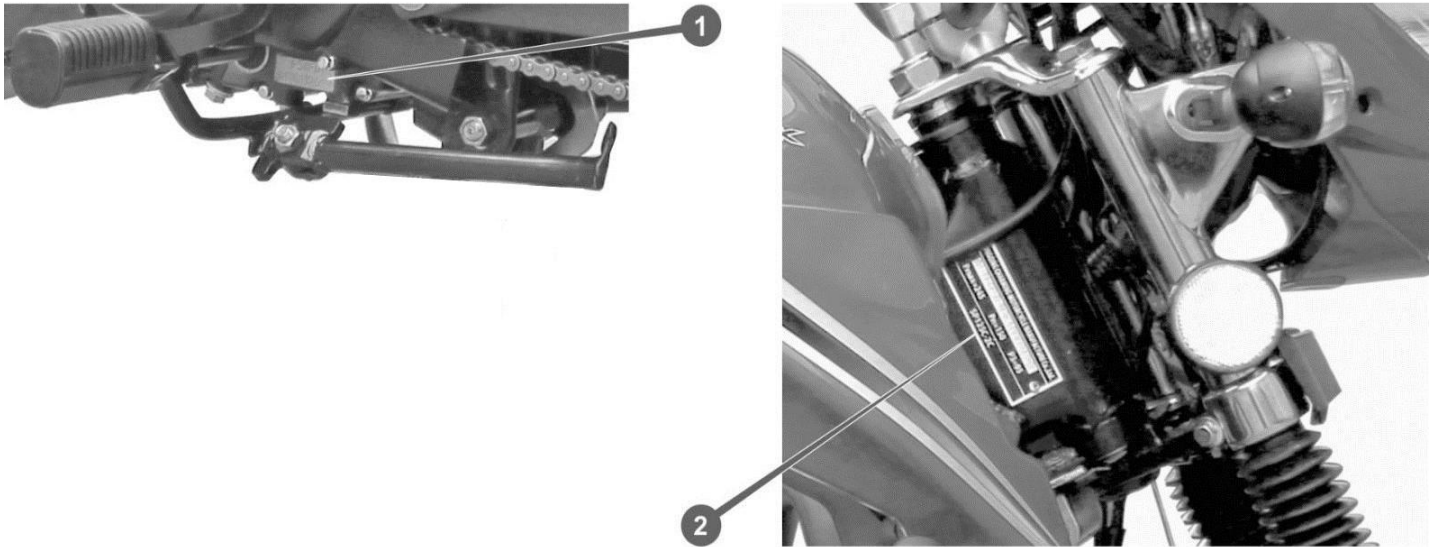
Рисунок 3.7. Розташування номера двигуна мотоцикла
