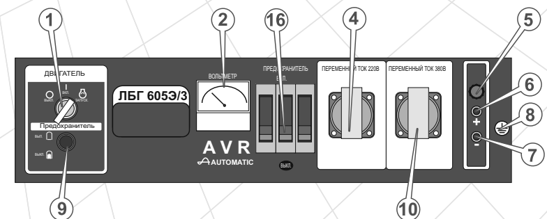
Панель управления ЛБГ-605Э/3
