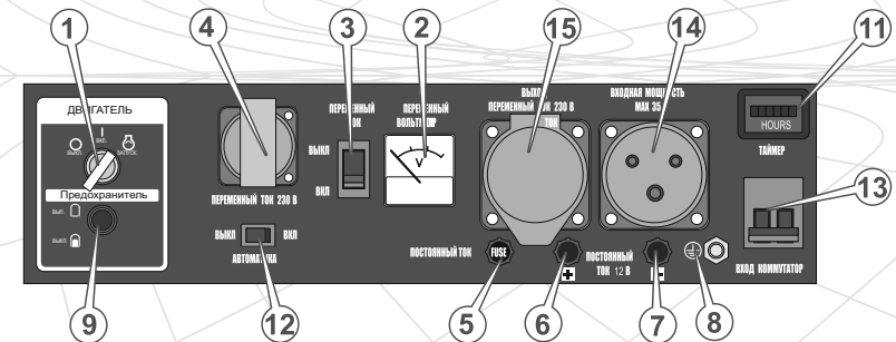
Панель управления ЛБГ-605Э/3
