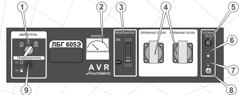
Панель управления ЛБГ-605ЭА
