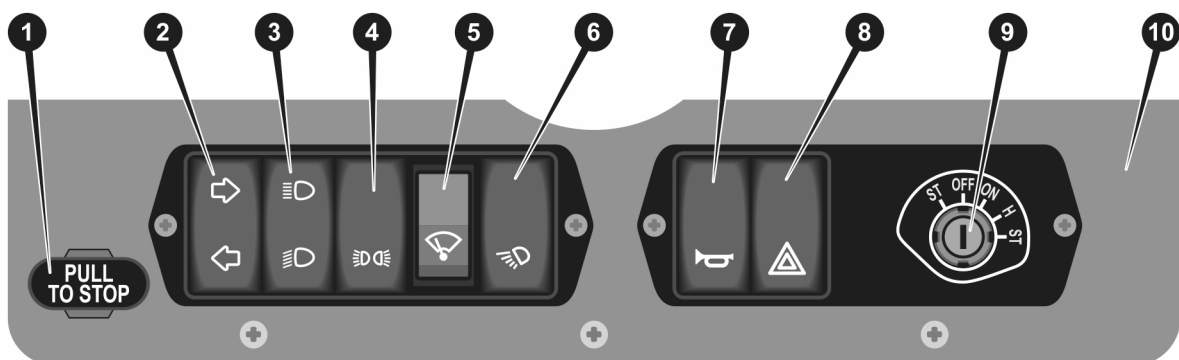
Малюнок 3.6. Лівий і правий блоки електроперемикачів
