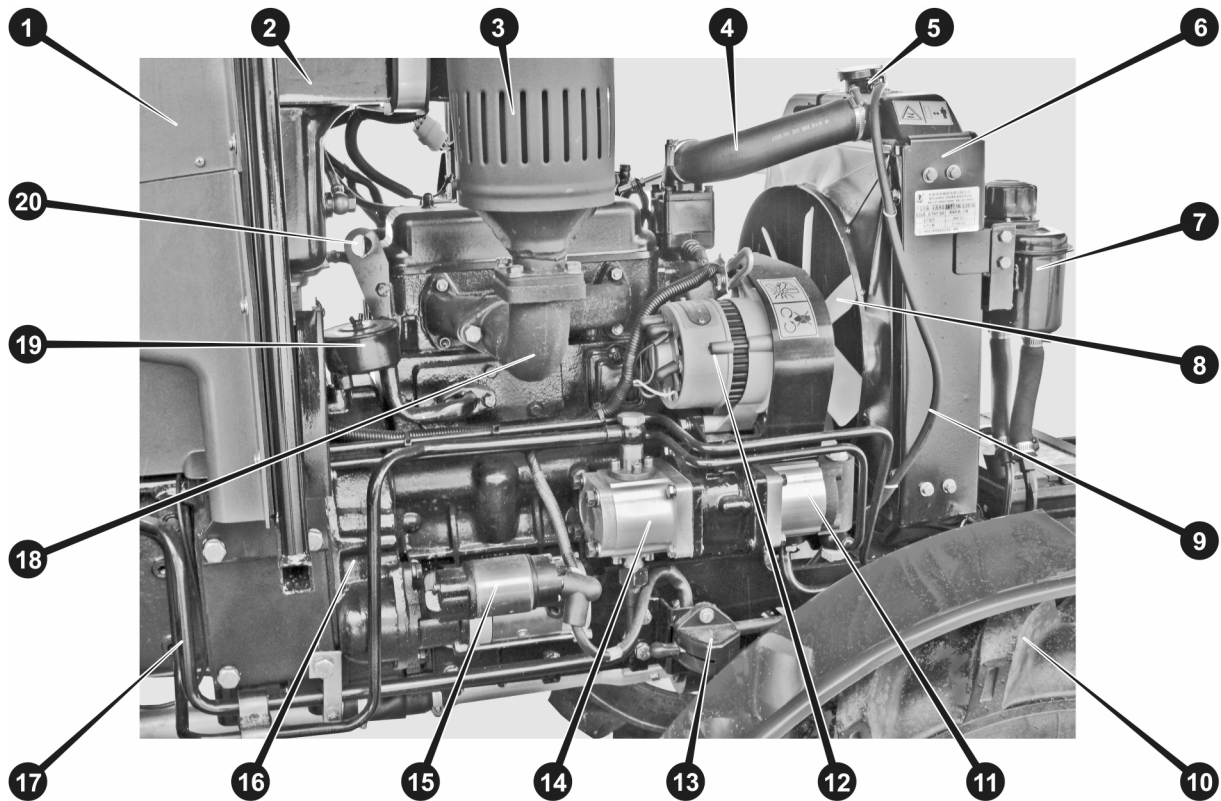
Рисунок 3.4. Двигун, вид справа
