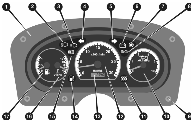
Рисунок 3.7. Електронна панель приладів
