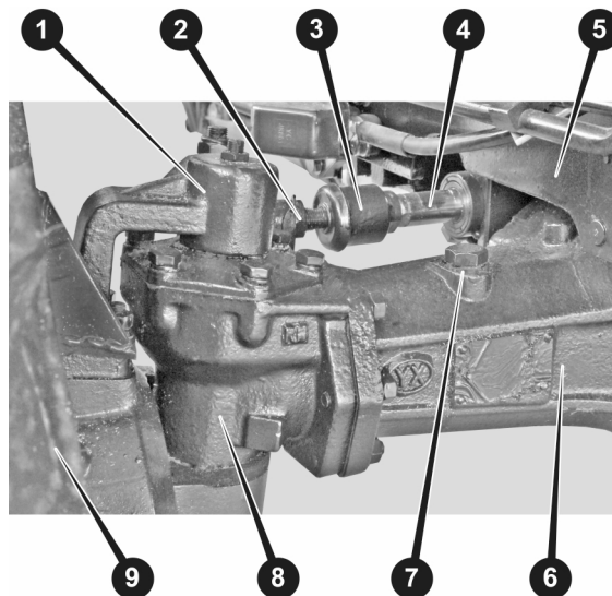
Рисунок 5.5. Регулювання сходження передніх коліс
