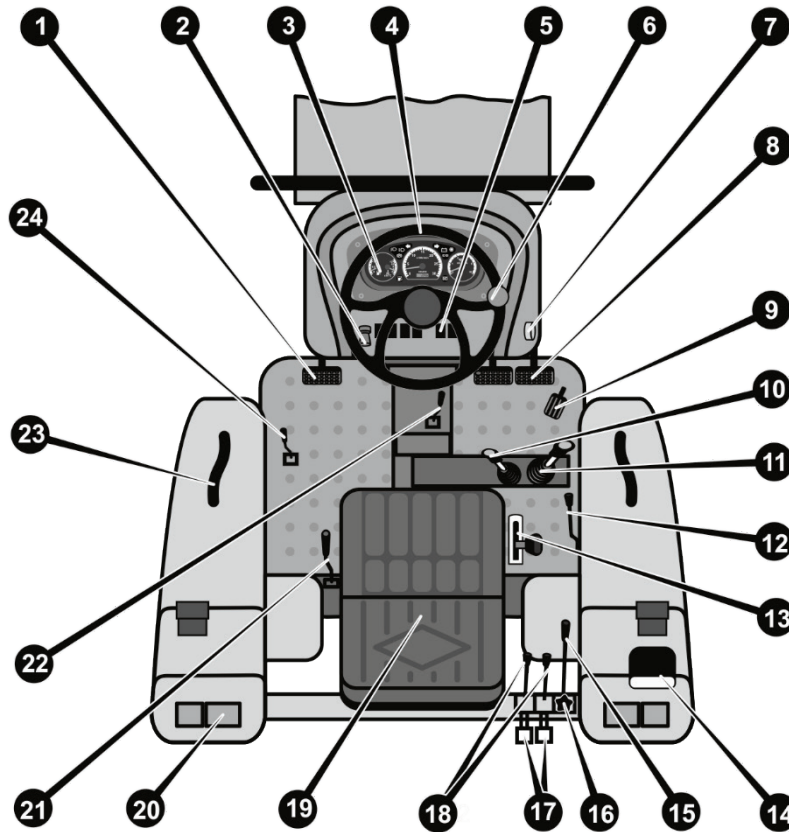
Рисунок 3.2. Схема розташування органів управління трактора Jinma 404HS
