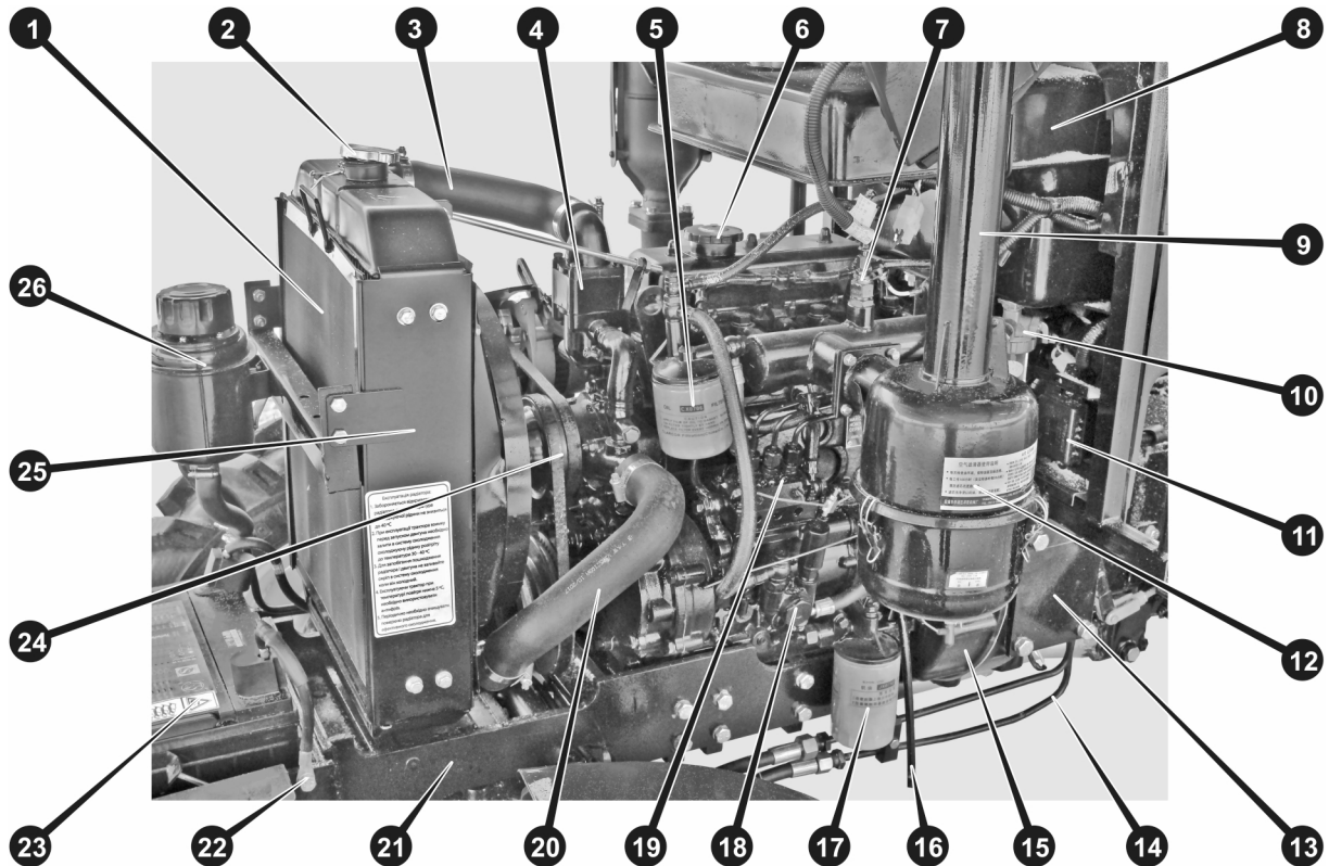
Рисунок 3.3. Двигун, вид зліва
