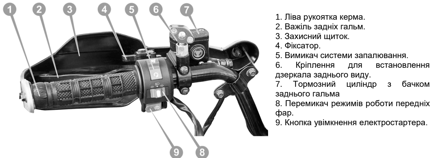
Рисунок 3.4. Блок перемикачів лівий
