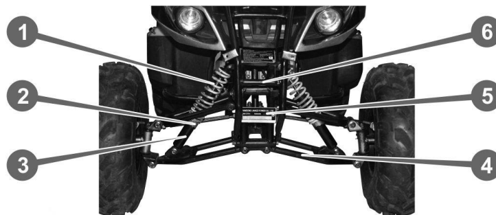
Рисунок 7.9. Передній міст
