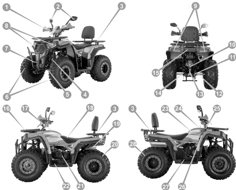
Рисунок 3.1.2 Розташування вузлів та агрегатів моделей SP200-3
