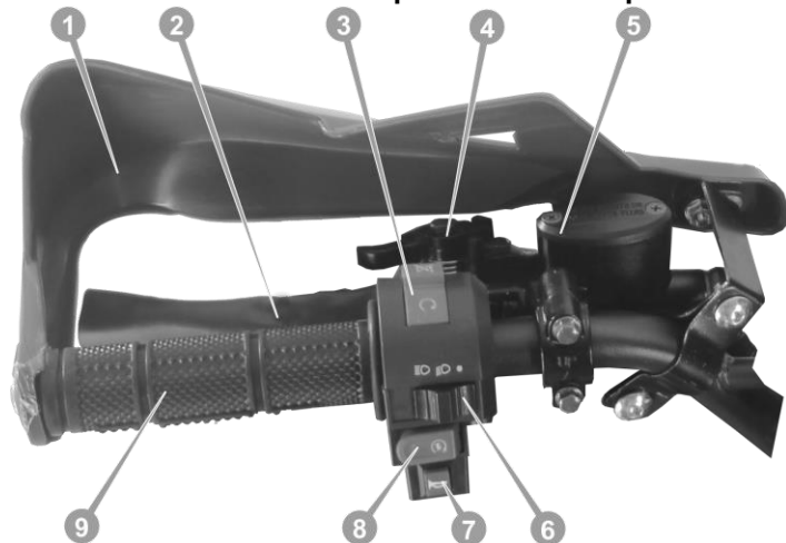
Рисунок 3.4.1. Блок перемикачів лівий моделей SP125-8, SP125-9, SP150-5
