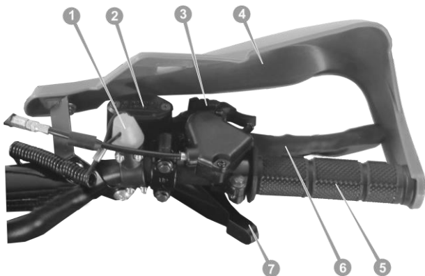
Рисунок 3.5.1. Блок перемикачів правий моделей SP125-8, SP125-9, SP150-5
