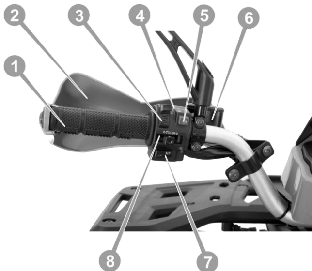
Рисунок 3.4.2. Блок перемикачів лівий моделі SP200-3
