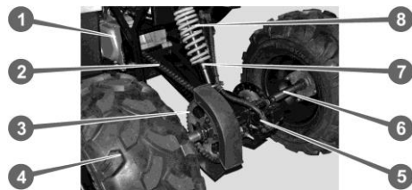
Рисунок 7.10. Задній міст
