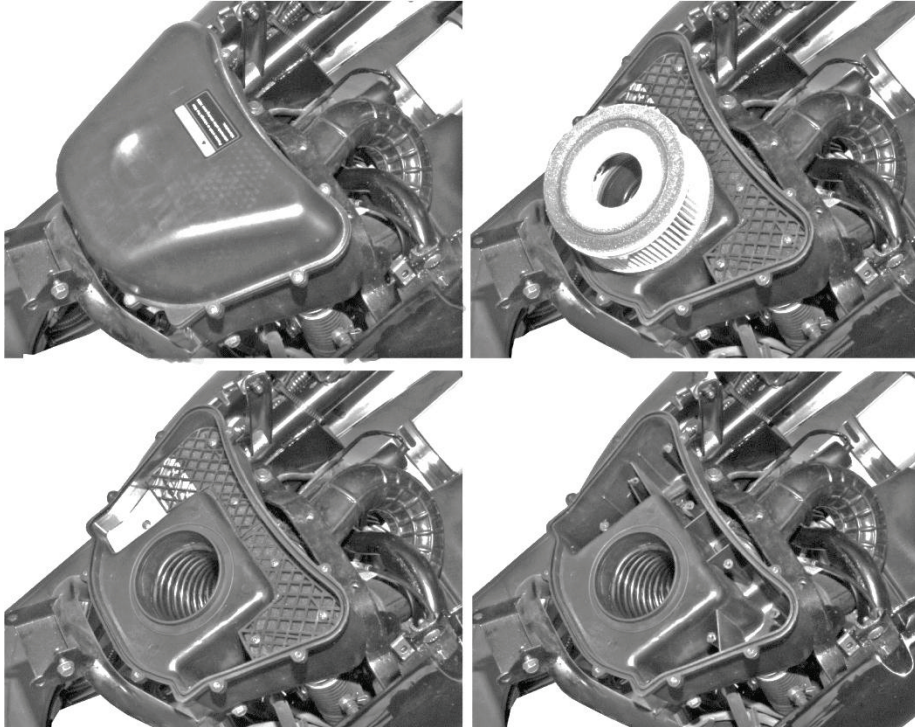
Рис. 6.6. Повітряний фільтр
