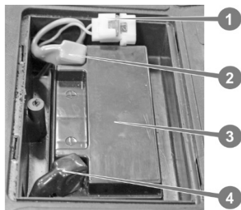
Рис. 5.5. Акумуляторна батарея
