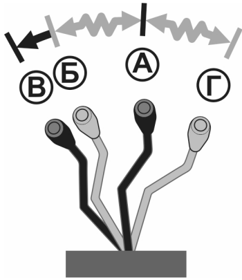
Рисунок 4.7. Положення важеля управління підйомником триточкової навісної системи
