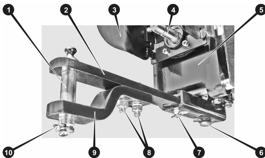
Рисунок 5.2. Тягово-зчіпний пристрій
