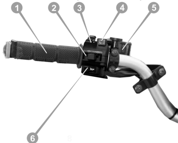
Рисунок 3.4. Блок перемикачів лівий
