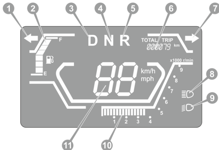
Рисунок 3.3 Панель приладів моделі SP125-15
