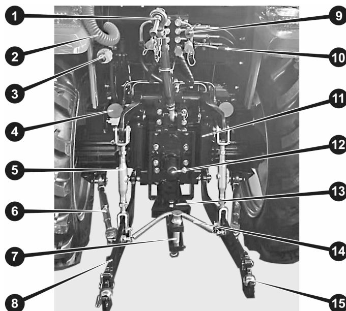
Рисунок 3.3. Триточкова гідронавісна система і вал відбору потужності
