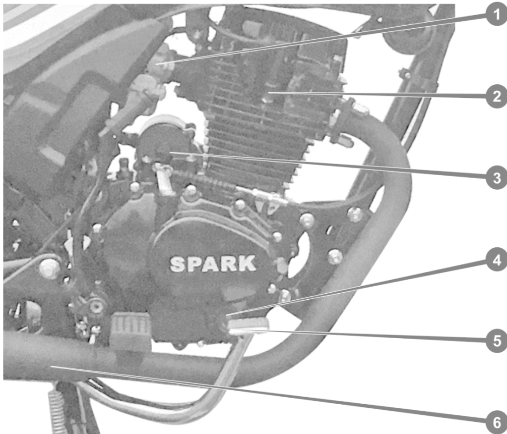
Рисунок 5. Вид двигуна праворуч
