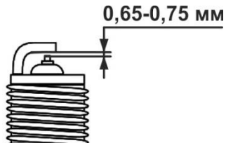
Рис. 11. Свічка запалювання, регулювання зазору.
