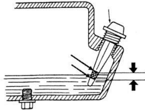
Рисунок 10. Перевірка рівня мастила у двигуні
