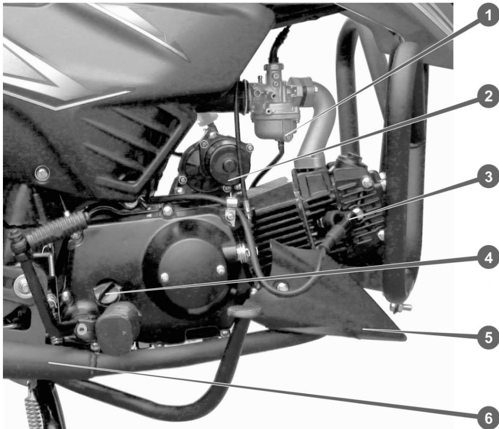
Рисунок 4. Вид двигуна праворуч
