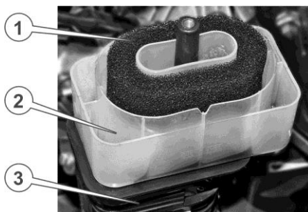
Рисунок 5.1. Повітряний фільтр
