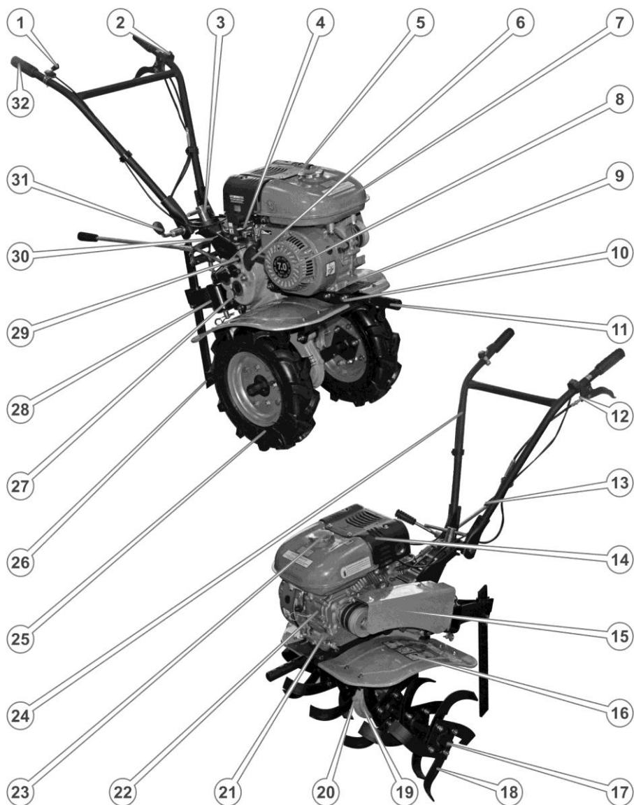
Рисунок 1.1. Елементи мотоблока
