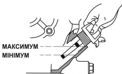
Рисунок 4.8. Пробка-щуп картера двигуна
